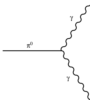
Fig. 1. Désintégration du pion neutre.
